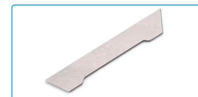
名称: 下刀(厚料) Description: Lower Knife (Heavy Duty) 代码/Part NO: 20119006 适配: E3-5×2-56 Machine Type: E3-5×2-56
