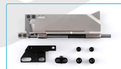
名称: 自动剪线组件 Description: No-Suction Trimmer Asm 代码/Part NO: 2071208200 适配: 900E/C3/C4 Machine Type: 900E/C3/C4
