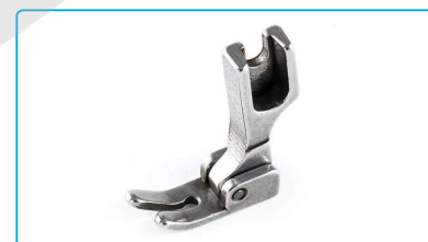
名称: P58N 全钢压脚 Description: Steel Presser Foot P58N 代 码/Part NO: 811305 适 配: 平缝机通用 Machine Type: All lockstitch machine series
