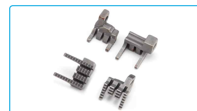
名称: 牙齿组件 Description: Feed Dog Assy 代码/Part No: 30714003 + 30714004 适配: 8670系列-01CB机型 Machine Type: 01CB type for 8670 series
