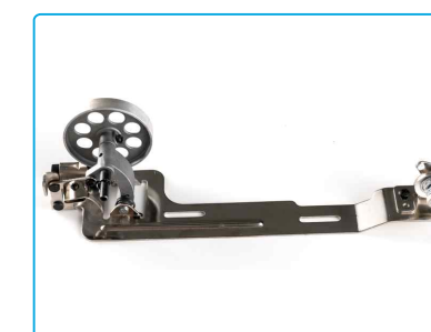
名称: 绕线器组件 Description: Bobbin Winder 代码/Part NO: 1013100600 适配: JK-8720 Machine Type: JK-8720
