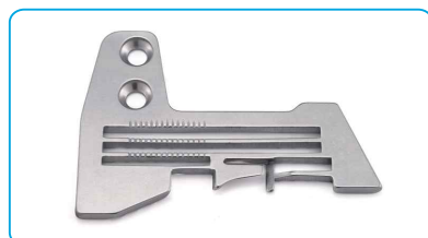
名称: 针板 Description: Needle Plate 代码/Part NO: 20115002 适配: E3-4-M2-24 Machine Type: E3-4-M2-24
