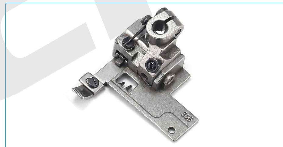
名称: 压脚(356) Description: Presser Foot (356) 代 码/Part NO: 30116005 适 配: W4/W4S/ K4/K5系列 02BB/23BB机型 Machine Type: 02BB/23BB type for W4/W4S/K4/K5 series
