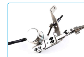
名称: 上切刀组件 + 电磁铁组件 Description: Upper Knife Holder Assembly 代码/Part No: 3013001600 + 3011900400 适配: 8670UT/K5S Machine Type: 8670UT/K5S
